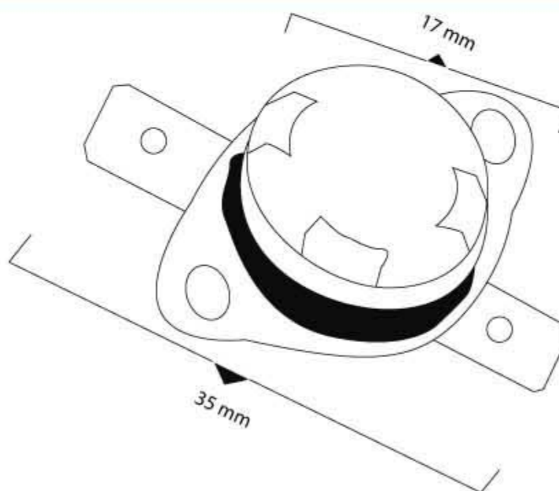
Sensor de temperatura del cabezal
