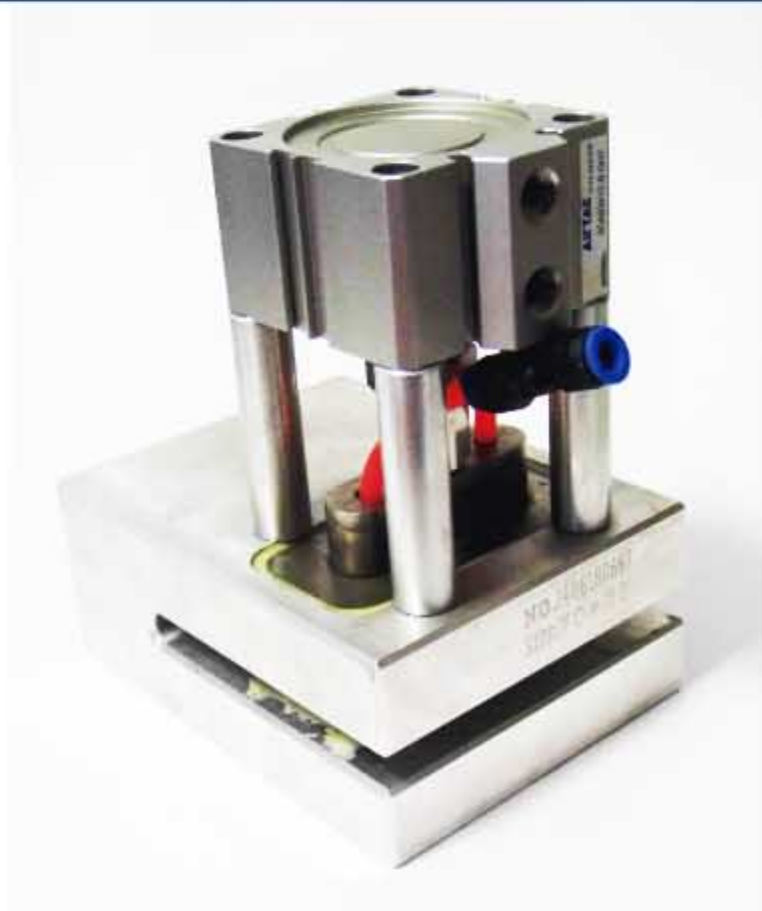
Troquel de Asa de 20 x 70
